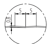
Szczegół A (2:1)
